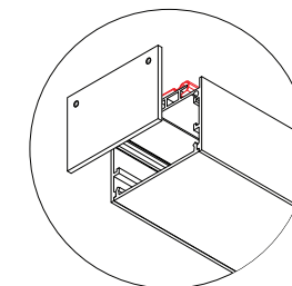
Detalhe do perfil aplicado no suporte de fixação
